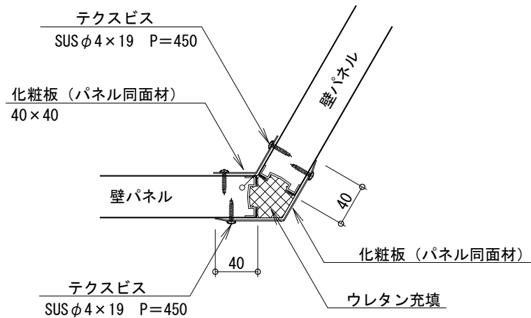
B部 (鈍角部) 詳細図
