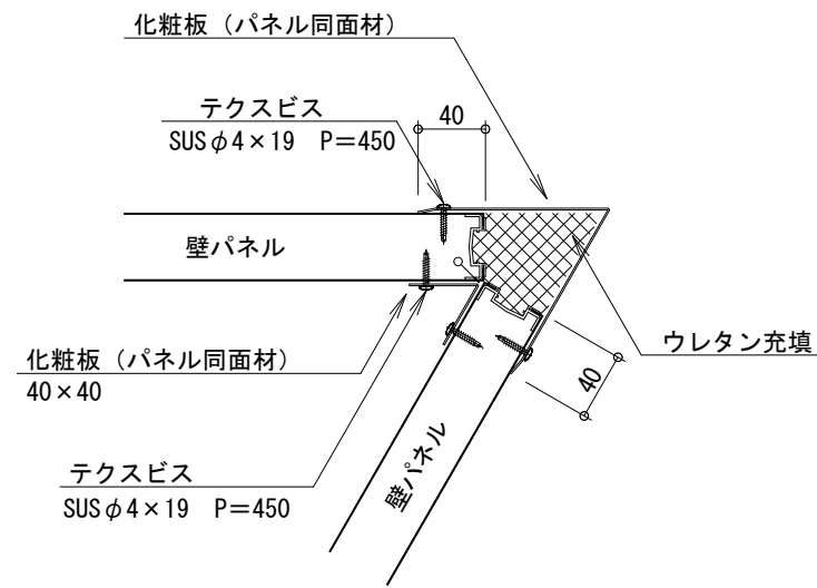
A部 (鋭角部) 詳細図
