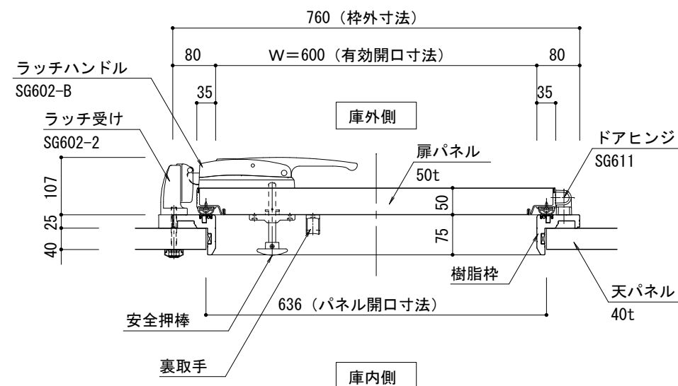
断面図 S=1/10
