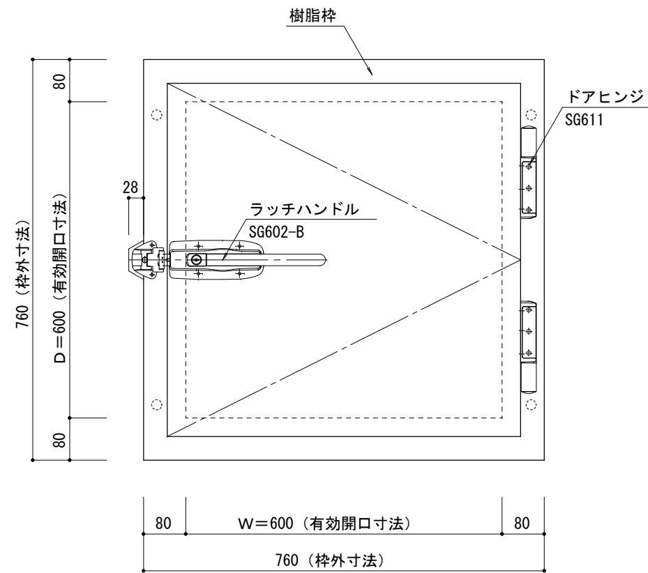
平面図 S=1/10
