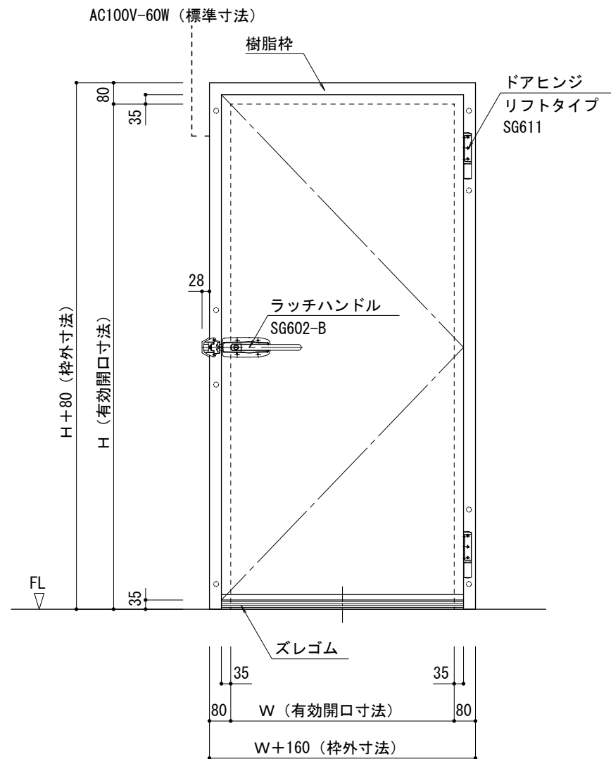
立面図 S=1/20
