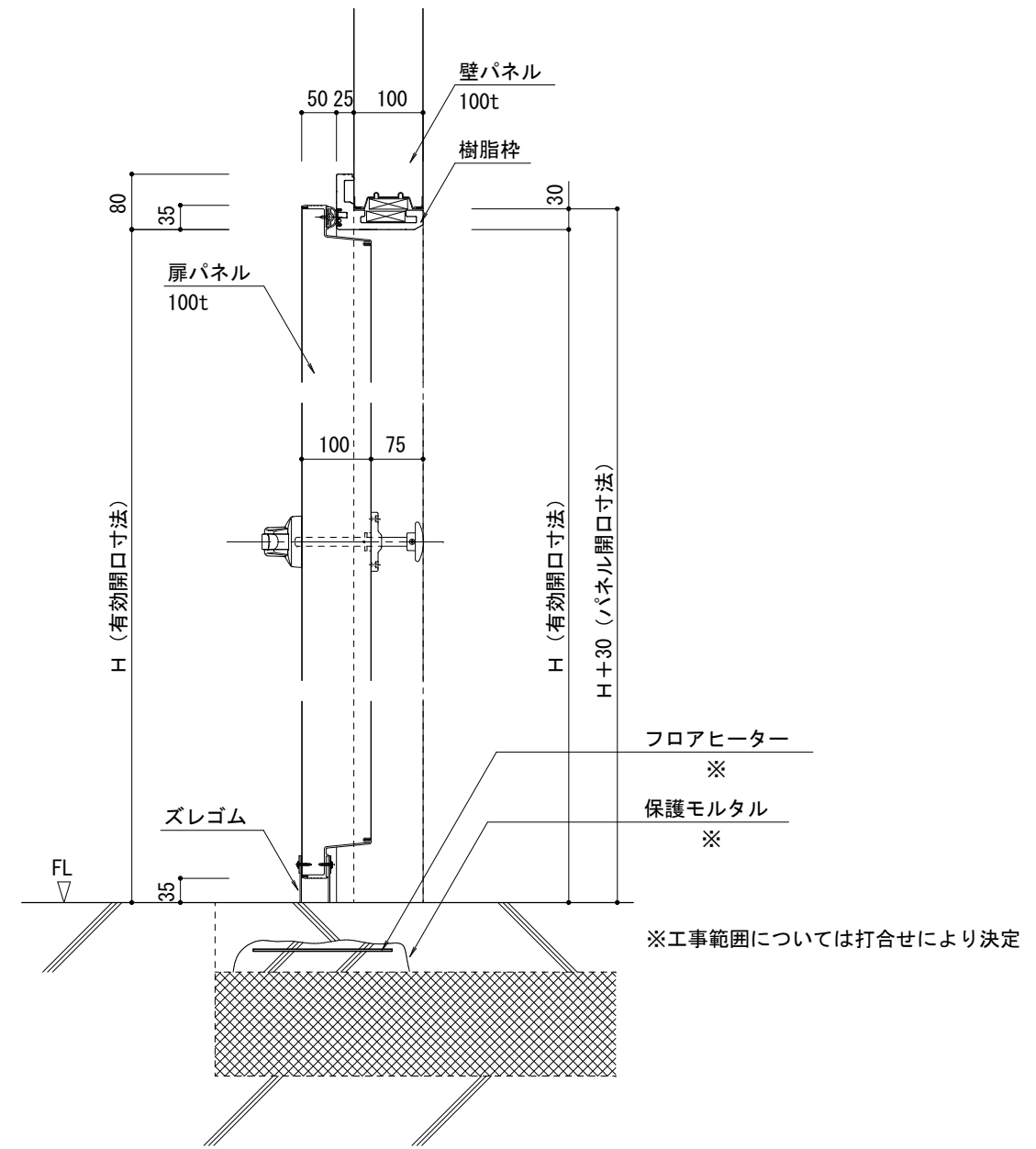
断面図 S=1/10
