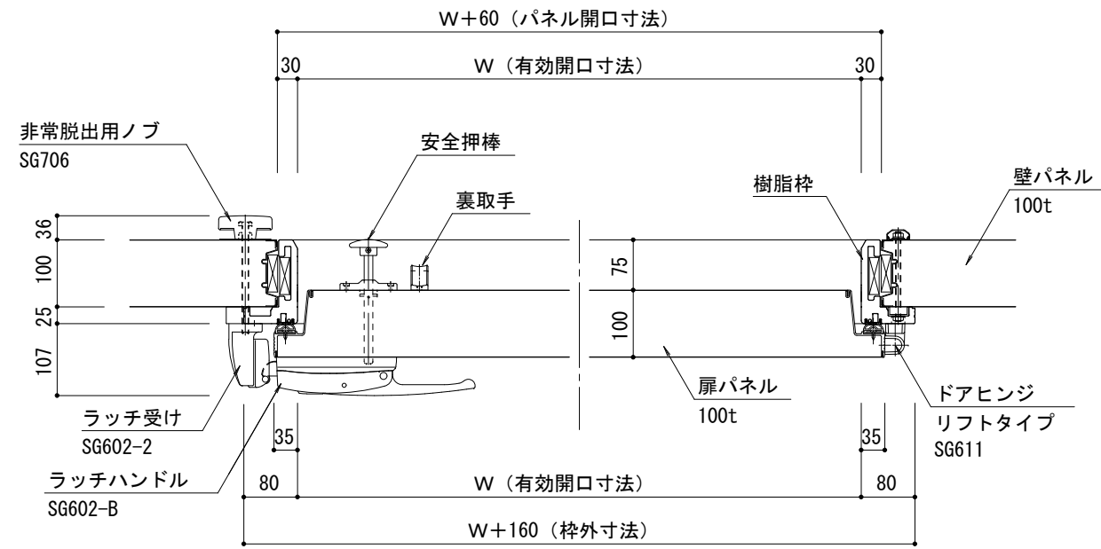
平面図 S=1/10
