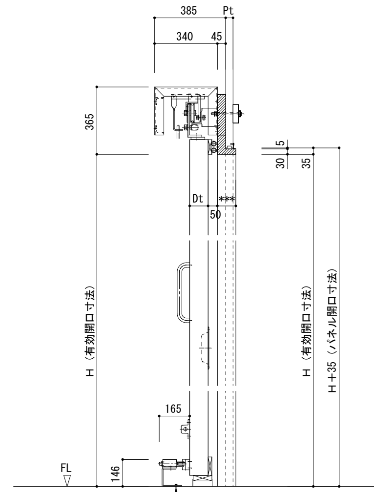
断面図 S=1/20
