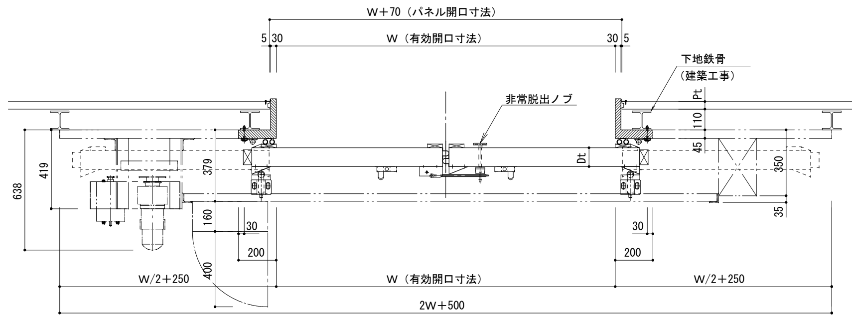
平面図 S=1/20
