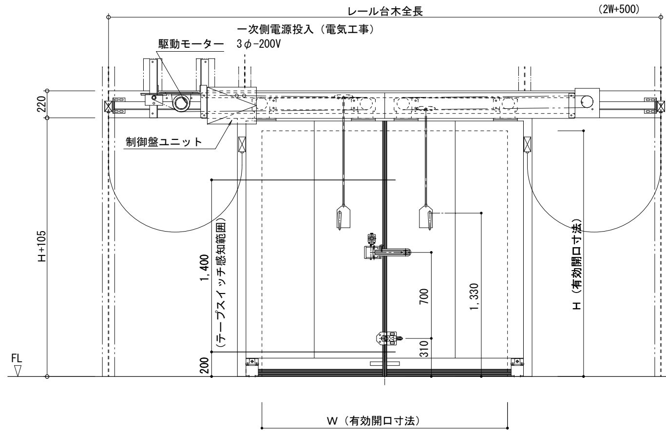
立面図 S=1/30
