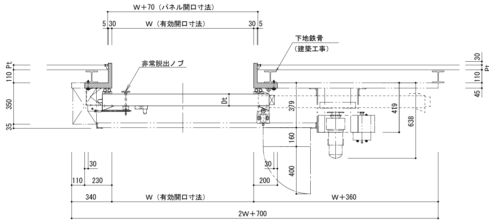
平面図 S=1/20
