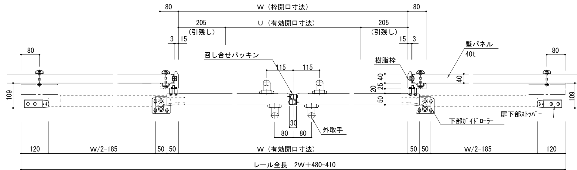
平面図 S=1/10
