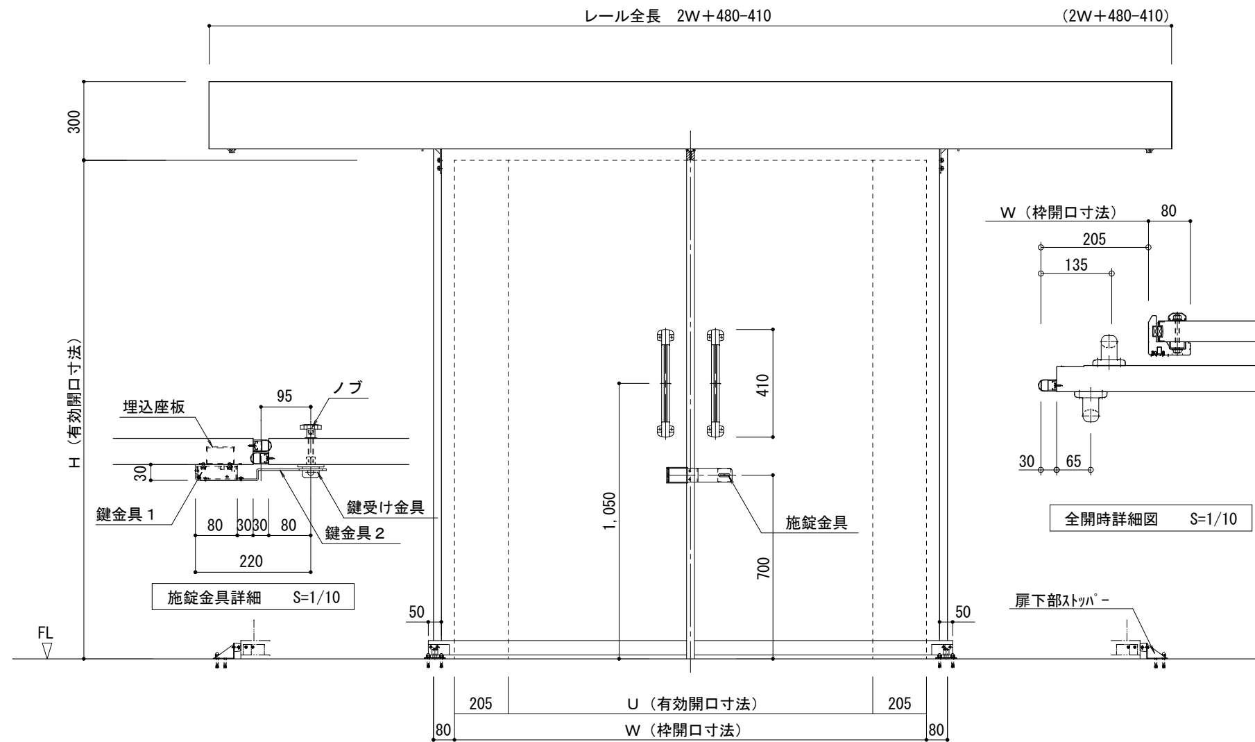
立面図 S=1/20
