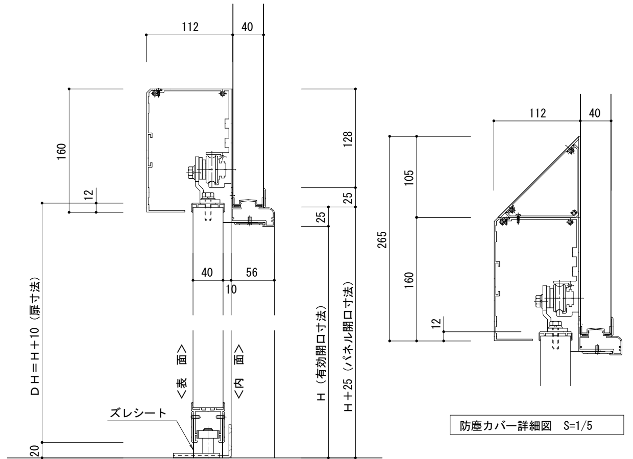
断面図 S=1/5
