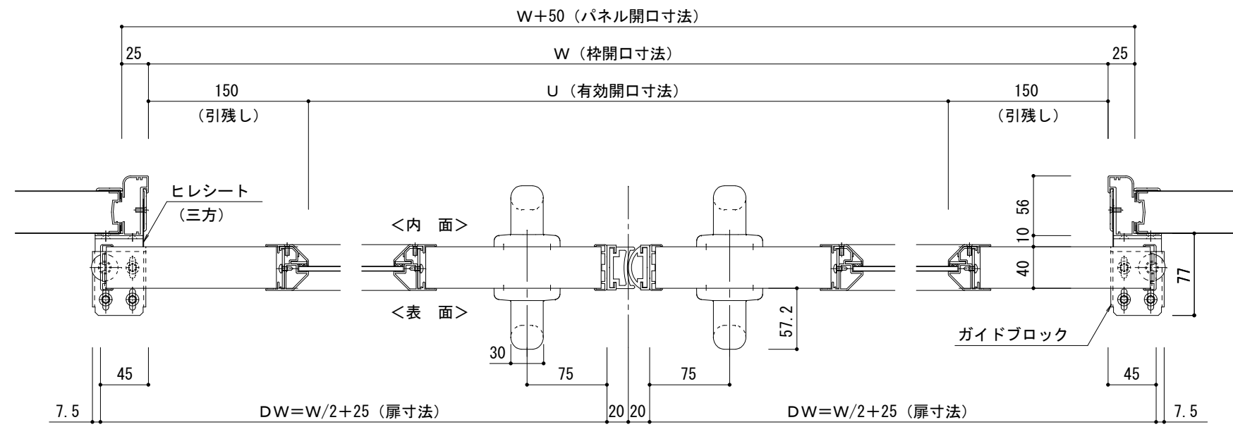
平面図 S=1/5
