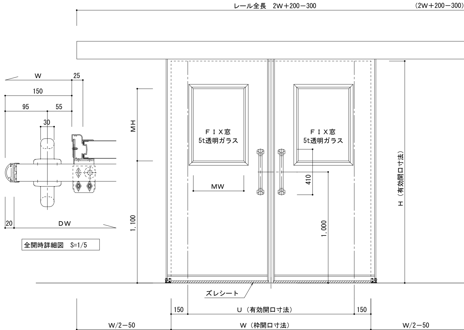
立面図 S=1/20
