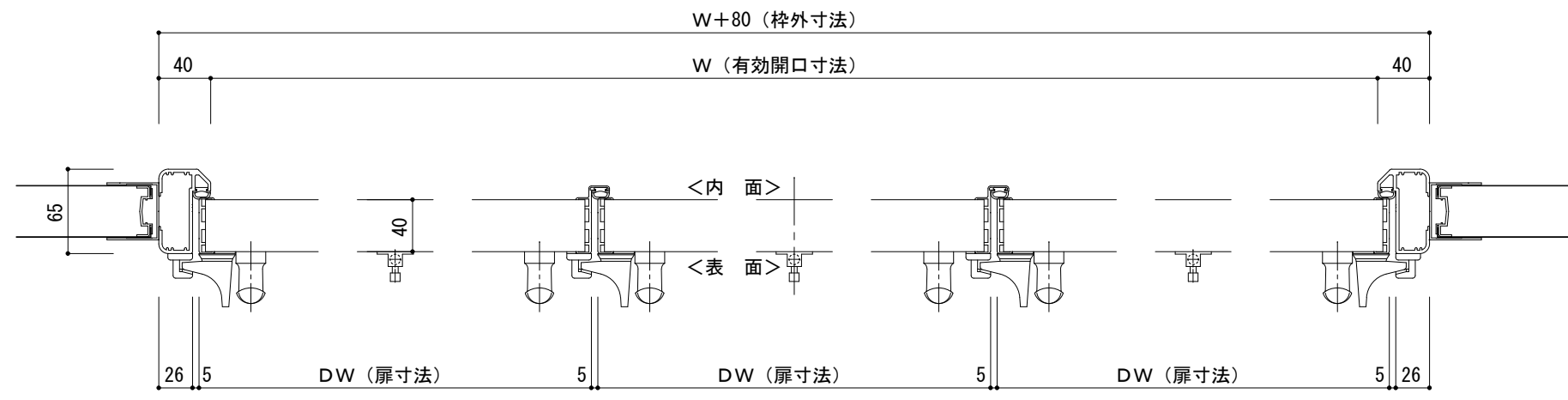
平面図 S=1/5
