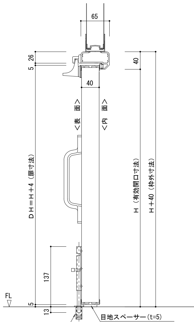
断面図 S=1/5
