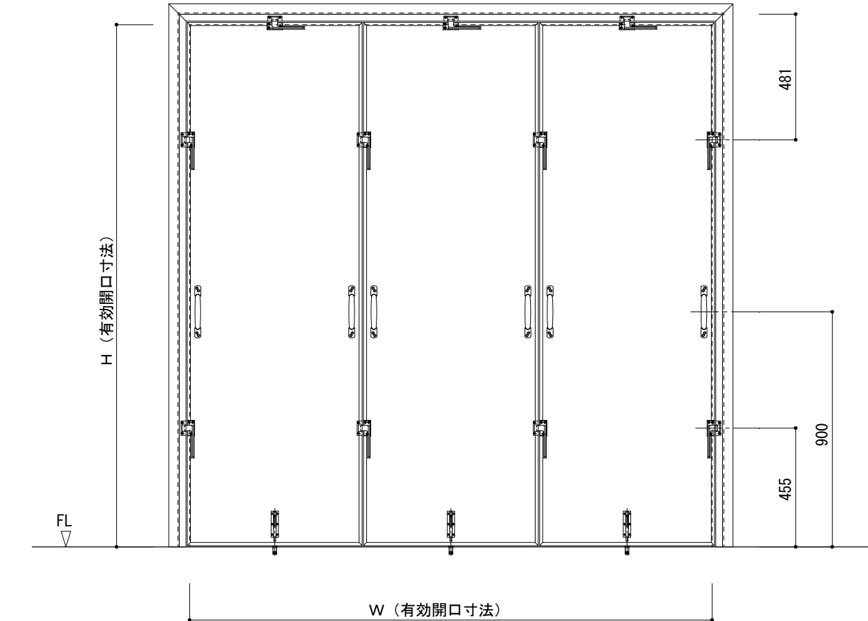
立面図 S=1/20
