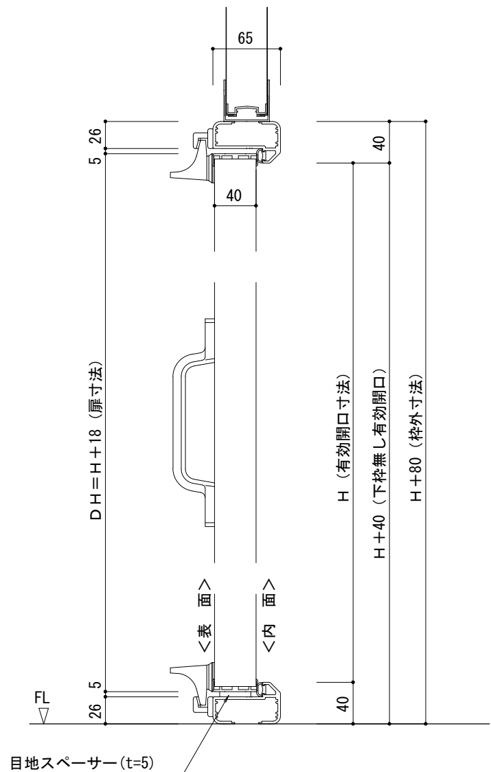
断面図 S=1/5
