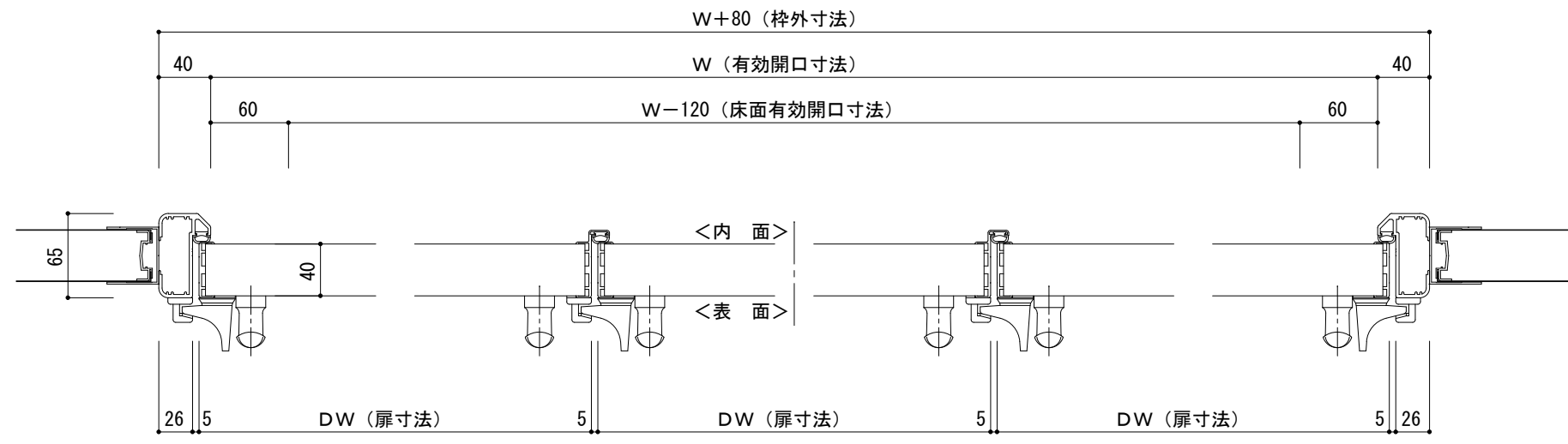
平面図 S=1/5
