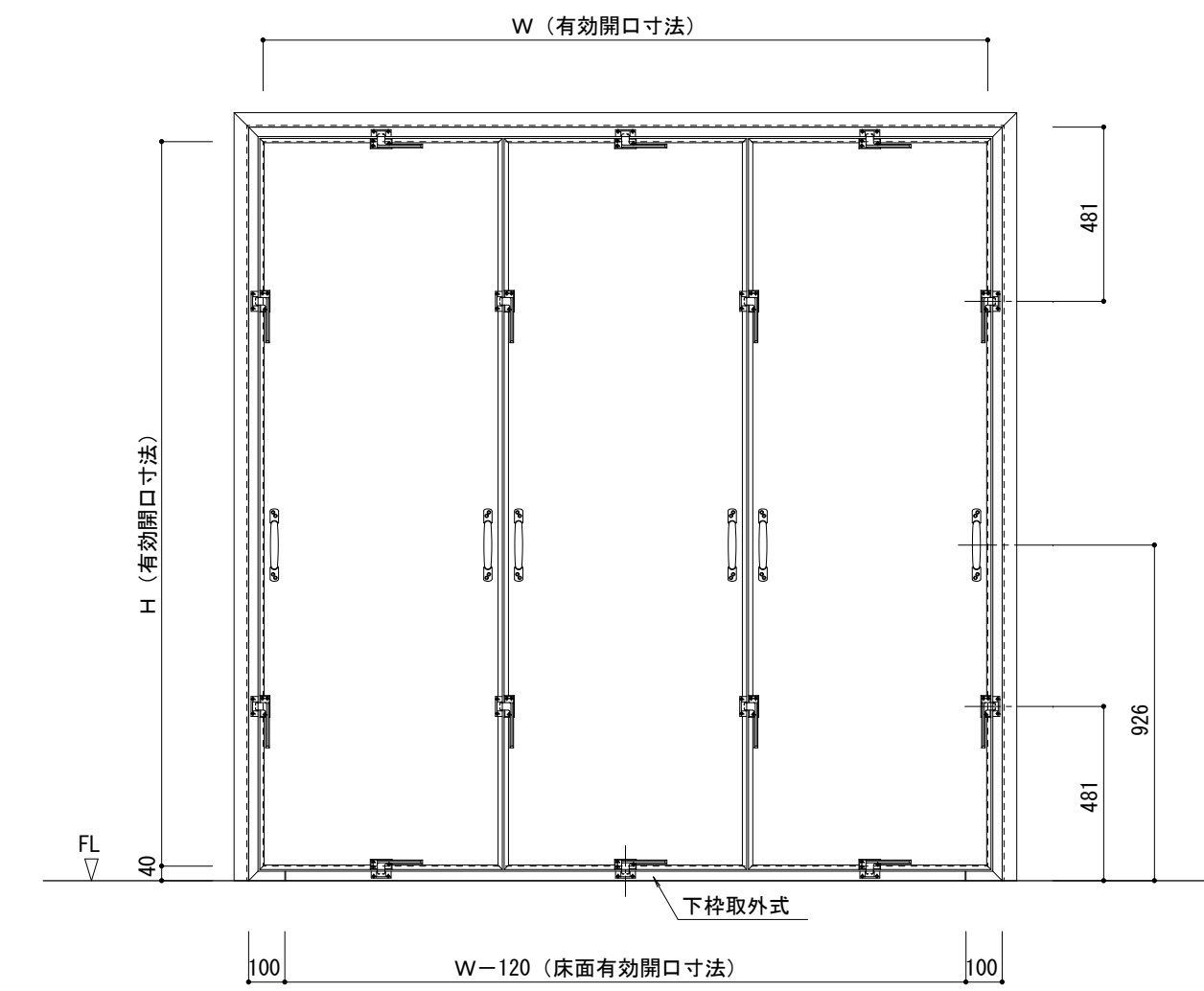
立面図 S=1/20
