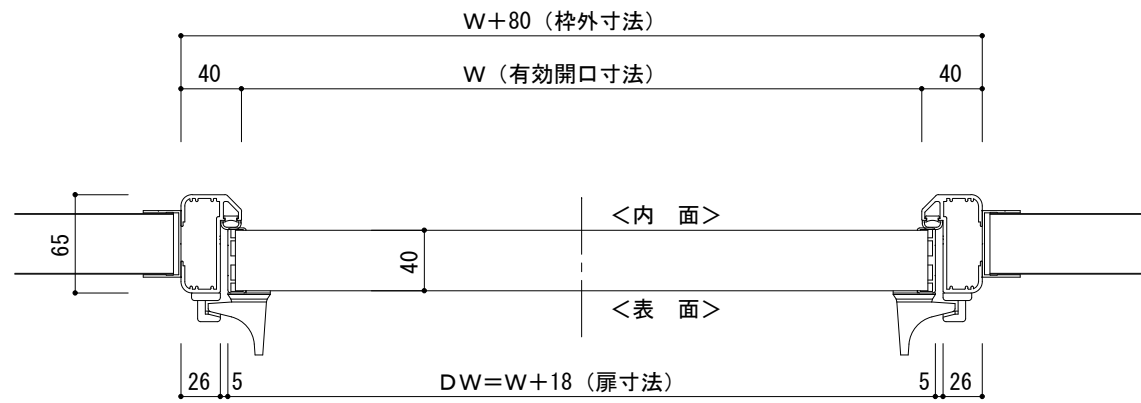
平面図 S=1/5
