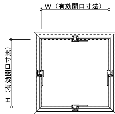
姿図 S=1/20
