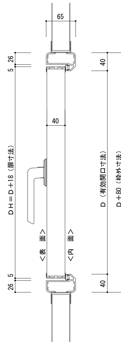
断面図 S=1/5
